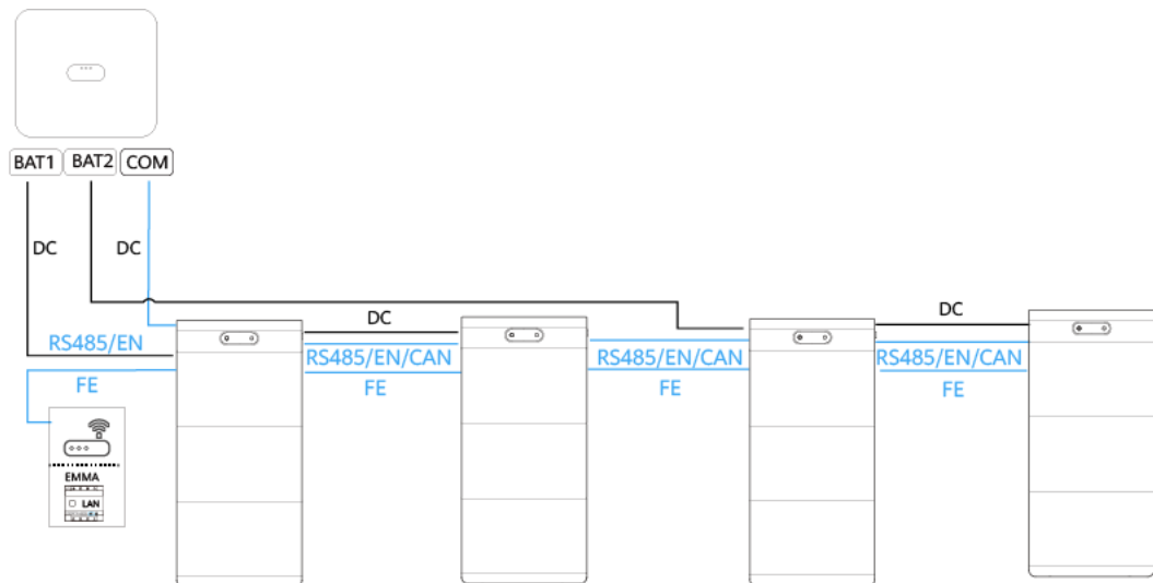
Figura 2-12 Conexión de los ESS al inversor (4)
