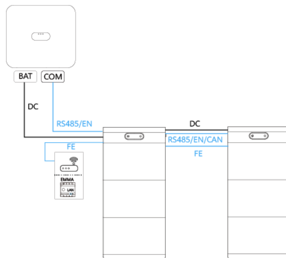
Figura 2-9 Conexión de los ESS al inversor (1)
