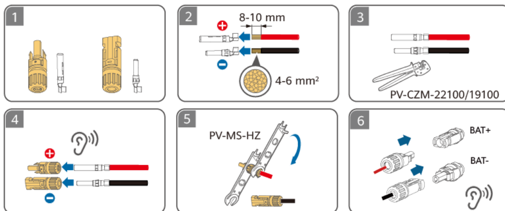
Figura 5-4 Conexión de los cables de entrada de CC
