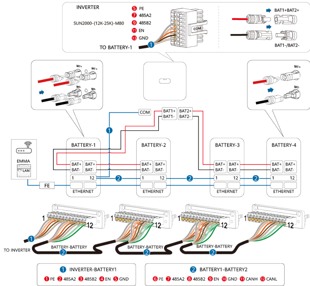
Figura 5-11 Inversor conectado a cuatro ESS
