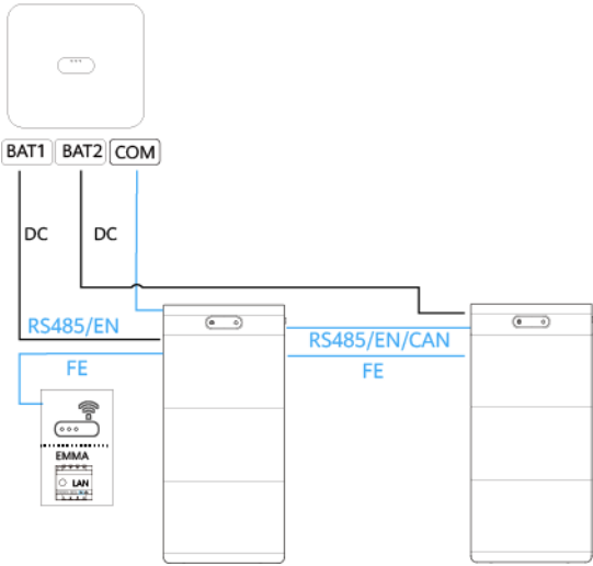
Figura 2-10 Conexión de los ESS al inversor (2)
