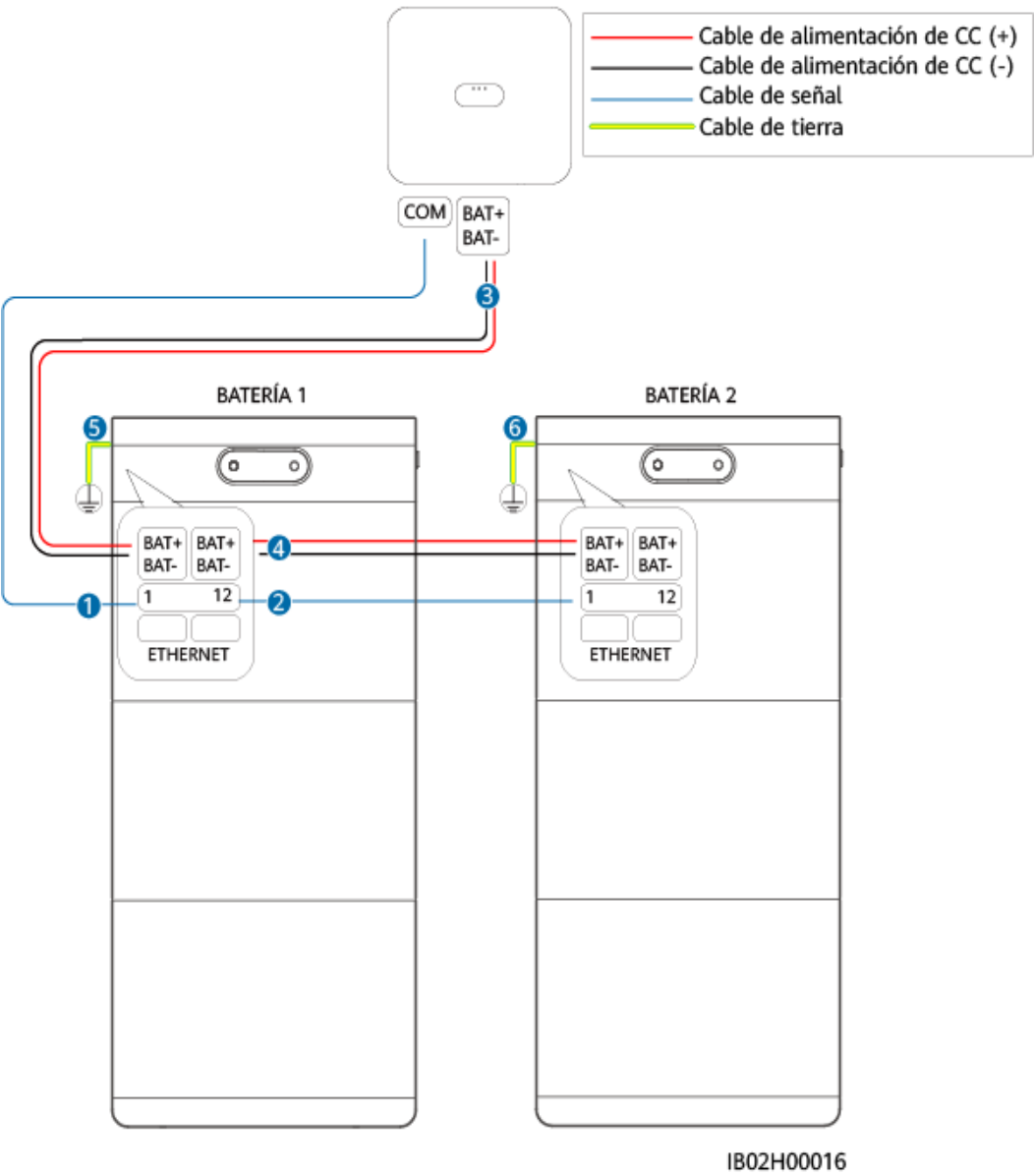
Figura 5-1 Conexiones de los cables del ESS
