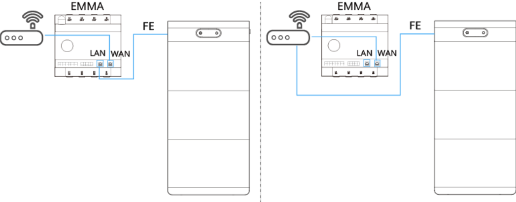
Figura 5-8 Puerto de red conectado al EMMA o al router
