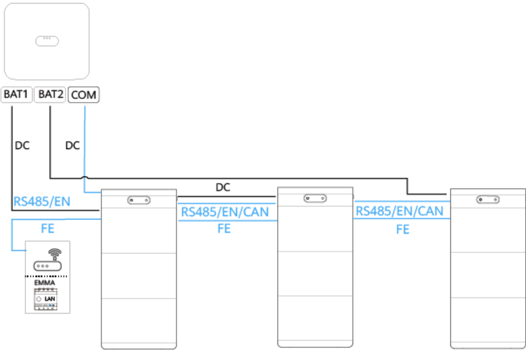
Figura 2-11 Conexión de los ESS al inversor (3)
