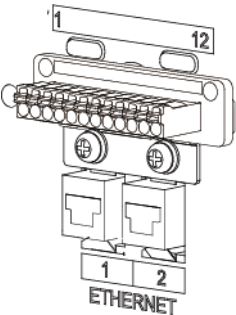
Figura 5-5 Puerto de señal
