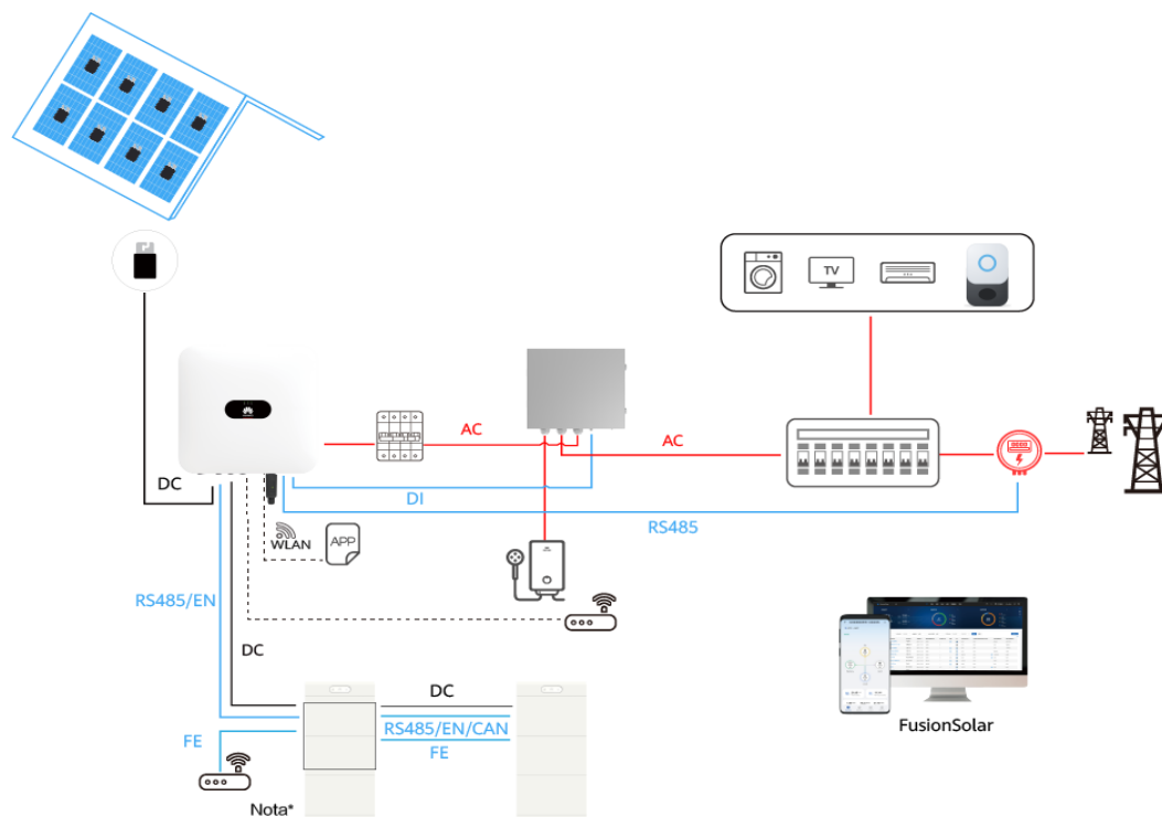
Figura 2-8 Escenario con/sin conexión a la red eléctrica
