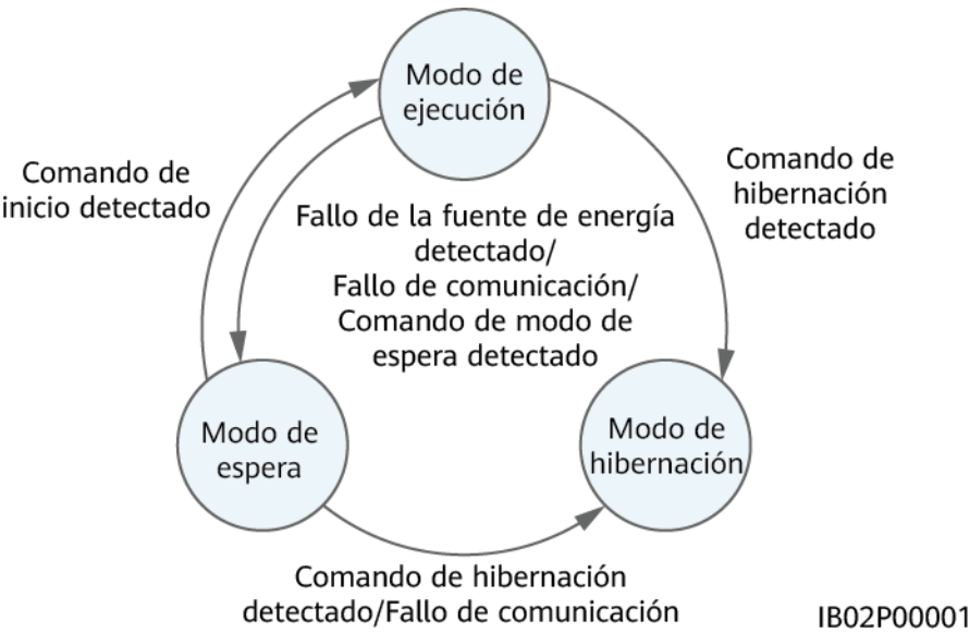
Figura 2-17 Cambio del modo de funcionamiento
