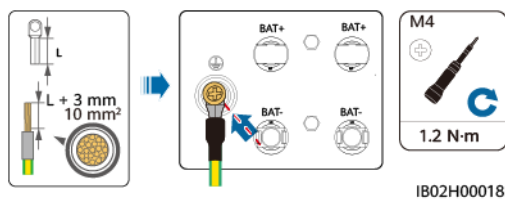
Figura 5-3 Conexión del cable de tierra
