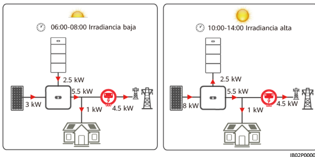
Figura 2-14 Totalmente proporcionada a la red
