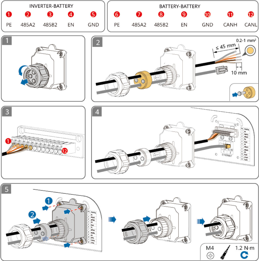
Figura 5-7 Conexiones de los puertos de señal
