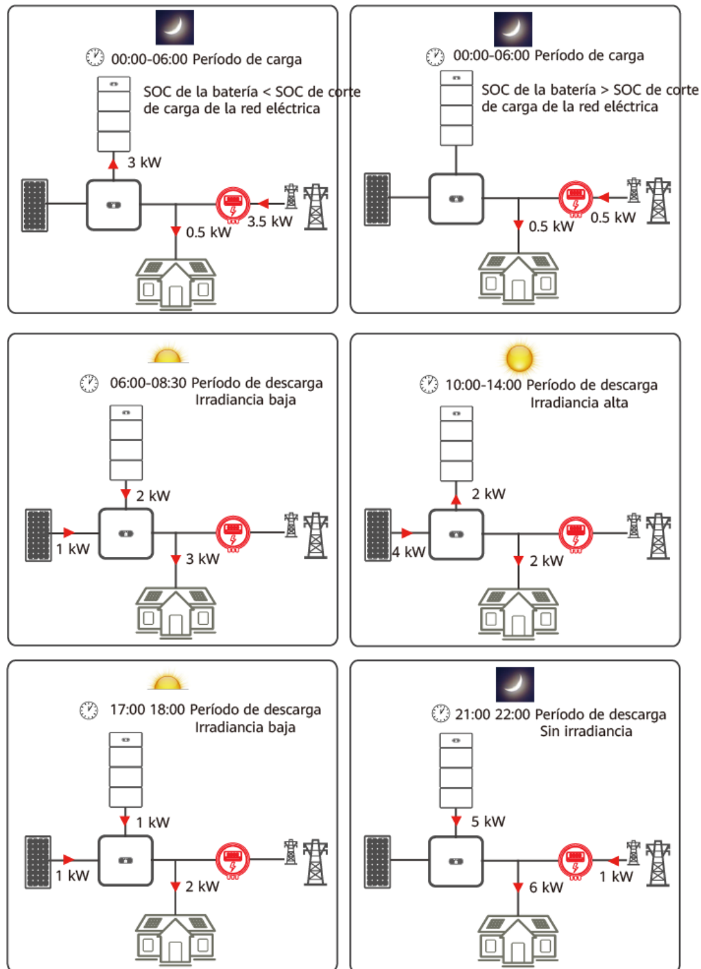
Figura 2-13 Ejemplo de TOU (carga de 00:00 a 06:00 y descarga de 06:00 a 24:00)
