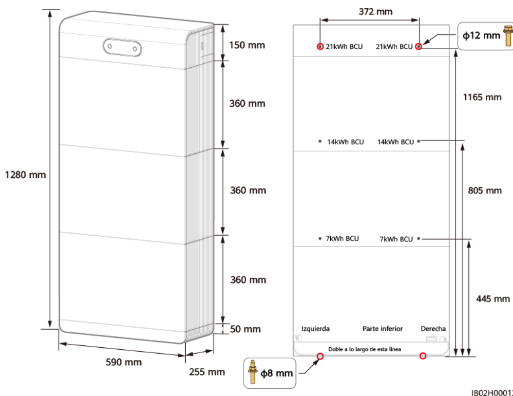
Figura 4-4 Dimensiones para el montaje en suelo
