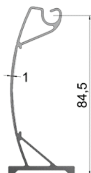
SOLEIRA (ALUMÍNIO) 0,723 Kg/m
