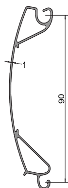
LÂMINA SIMPLES (ALUMÍNIO) 0,593 Kg/m
