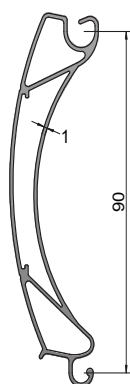
LÂMINA DUPLA (ALUMÍNIO) 0,784 Kg/m
