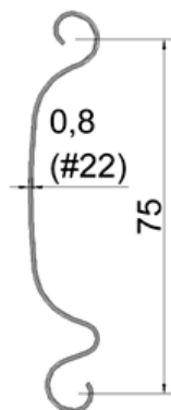
LÂMINAS DE AÇO 0,788 Kg/m
