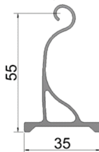
SOLEIRA DE ALUMÍNIO PARA LÂMINAS DE AÇO 0,581 Kg/m
