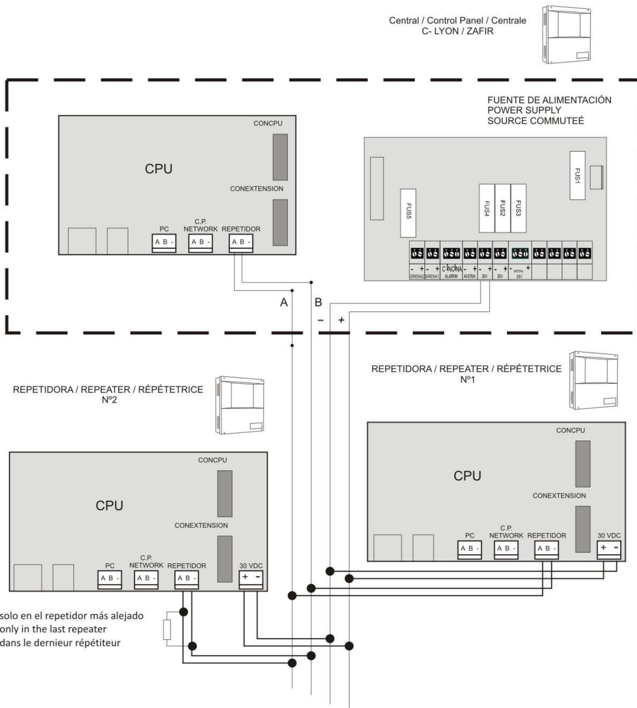
Figura 16. Conexión repetidores
