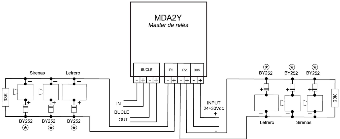
Figura 6. Esquema conexionado MDA2Y
