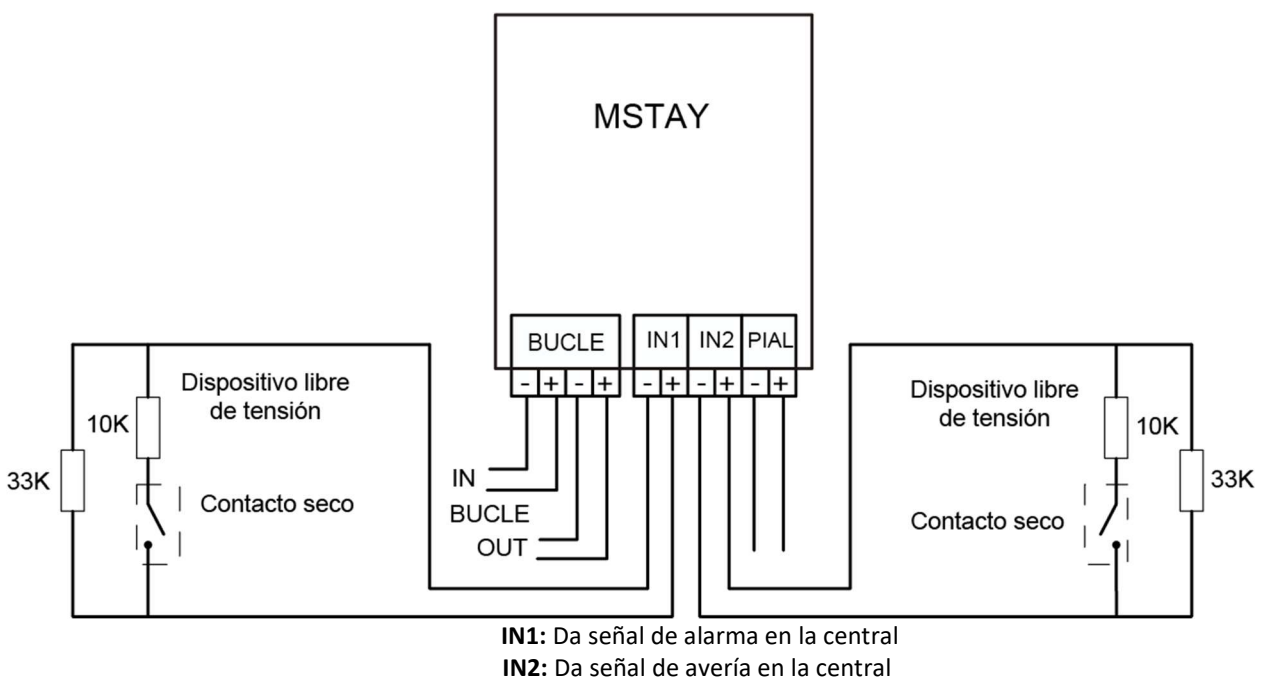
Figura 4. Esquema conexionado MSTAY
