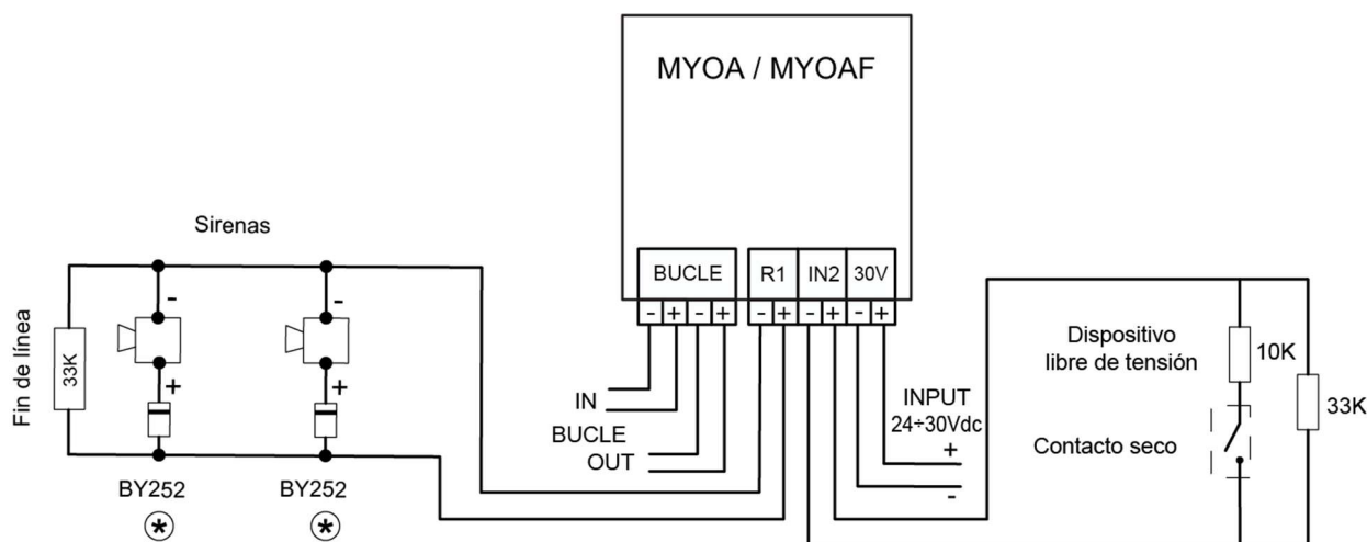
Figura 5. Esquema conexionado MYOA
