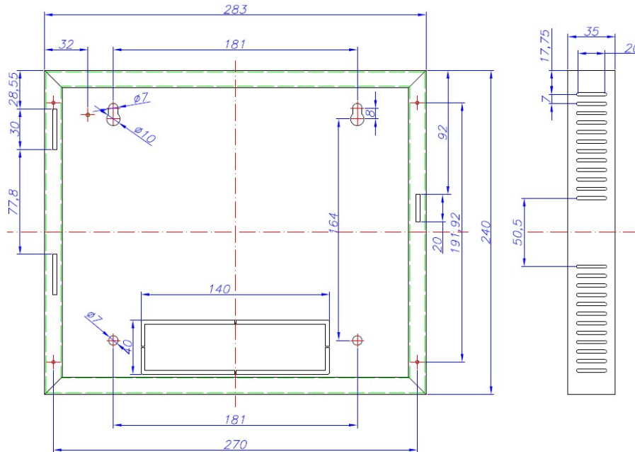
Figura 15. Cofre repetidor
