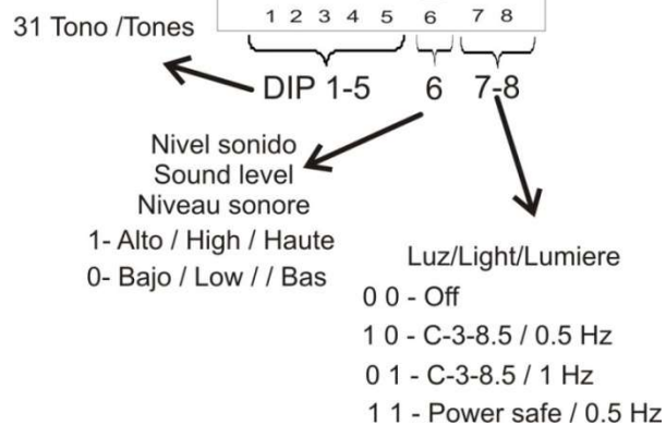
Figura 14C. Configuración DIP A50ZSLDR
