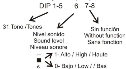
Figura 14B Configuración DIP A50ZSDDR
