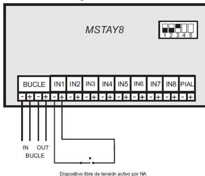
Figura 10. Esquema conexionado MSATY8
