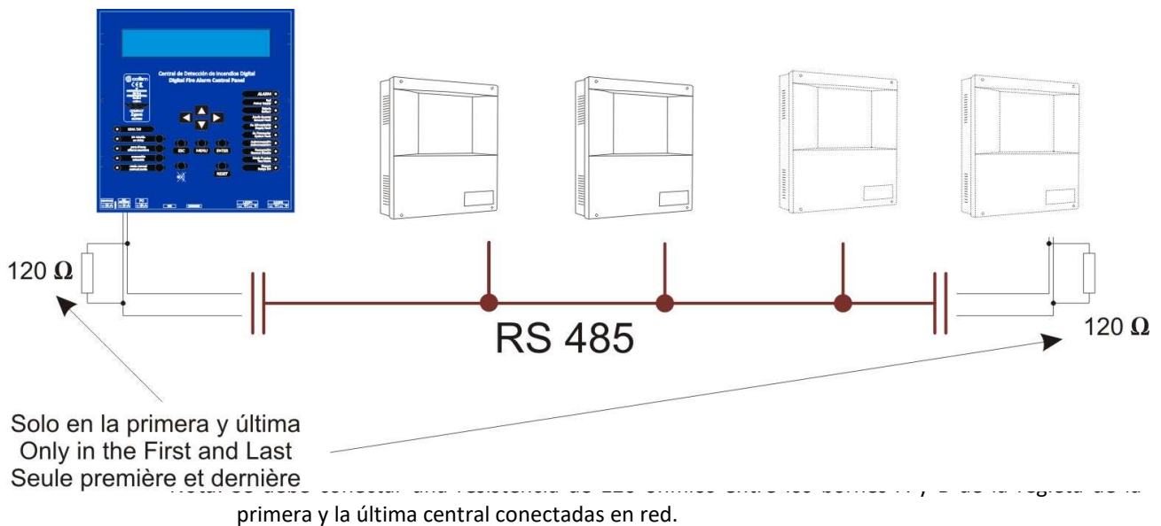
Figura 18. Conexión red de centrales
