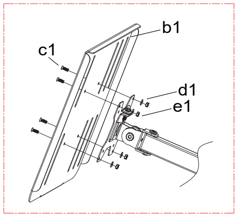
Ajuste y apriete el perno con la Llave Allen suministrada (i) para fijar el ángulo de inclinación.
