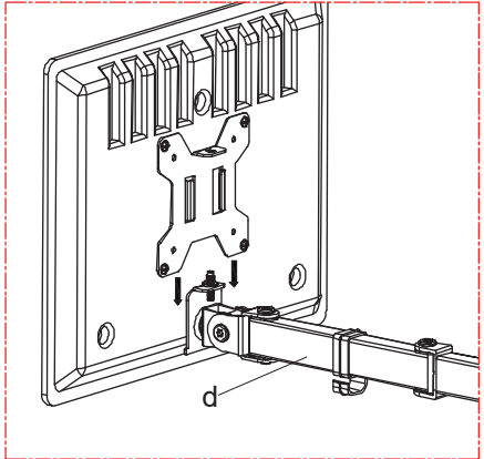
Inserte el monitor en la cabeza. del brazo giratorio.
