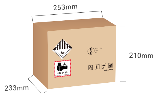
1* UN Carton
